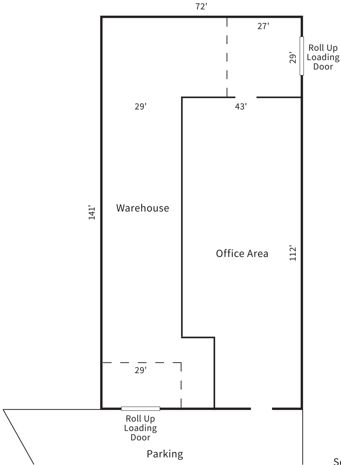
UNIT 101 SITE PLAN
